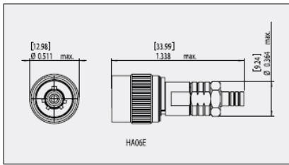
HA06E-*-*-* Plug
