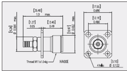
HA00E-*-*-* Receptacle
