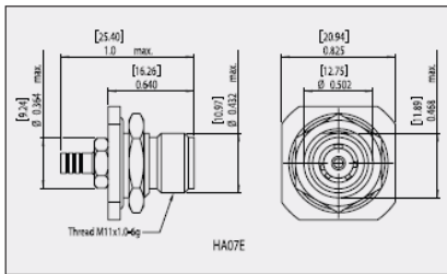
HA07E-*-*-* Jam Nut Receptacle
