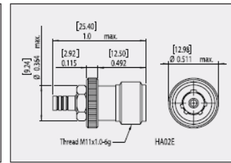
HA02E-*-*-* Free Receptacle
